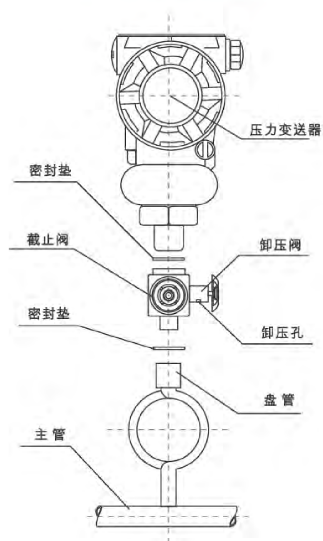
图4 安装简图
