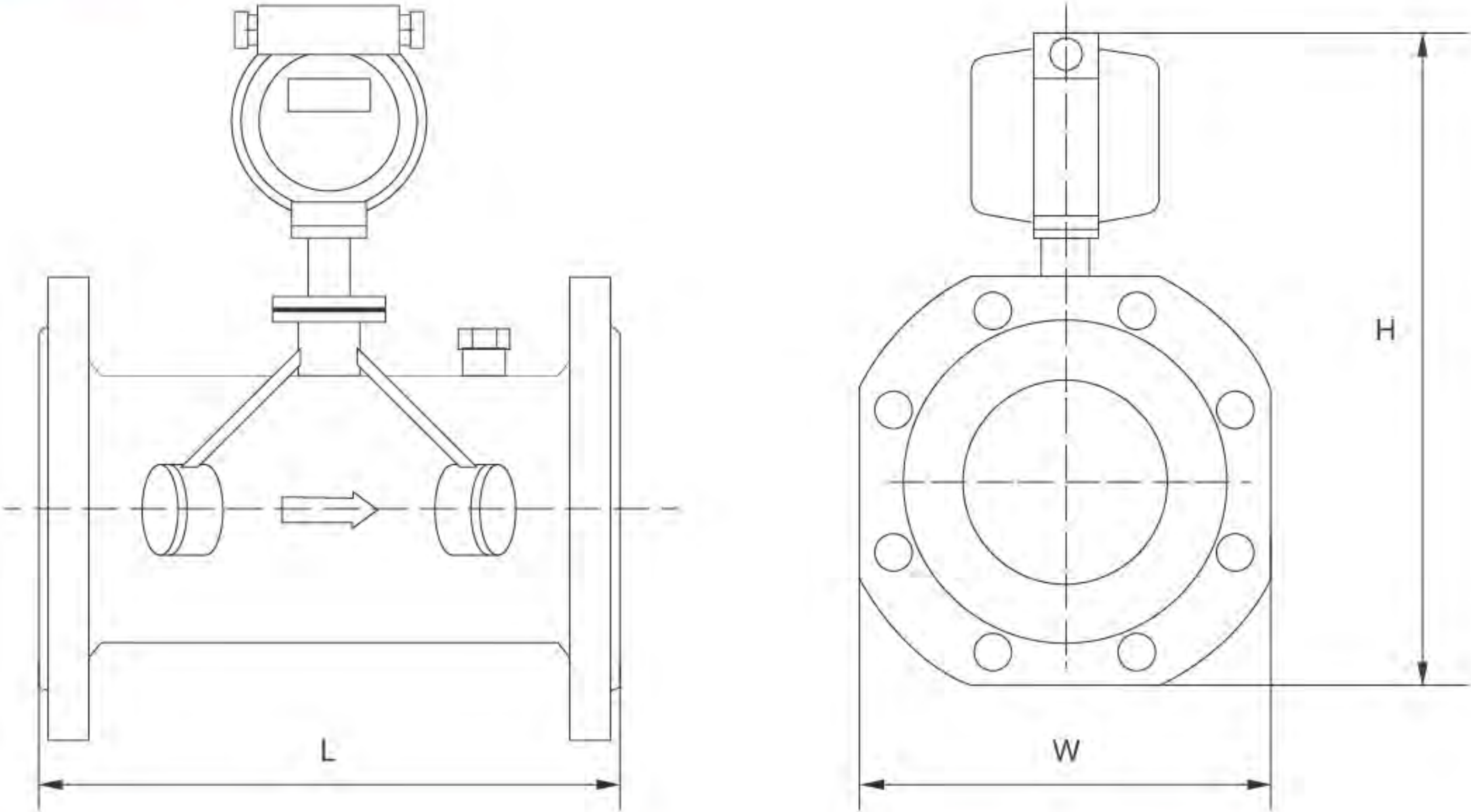
» 尺寸示意图
