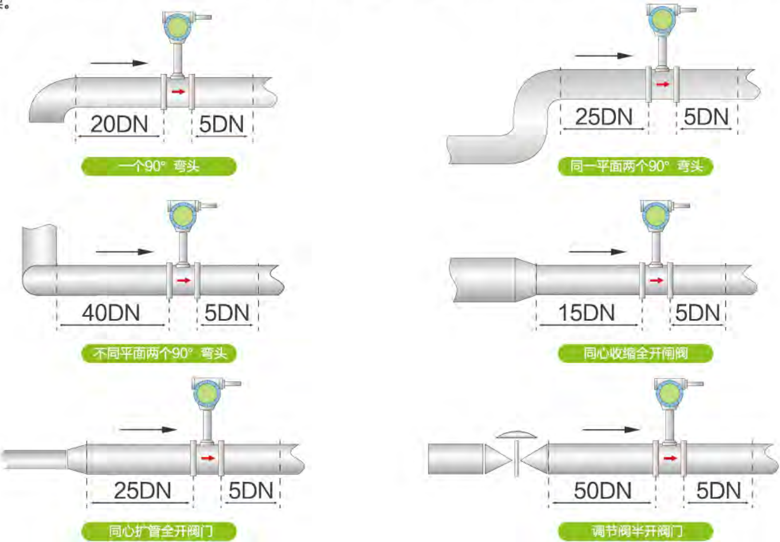
图二 流量计上、下游直管段长度的要求
