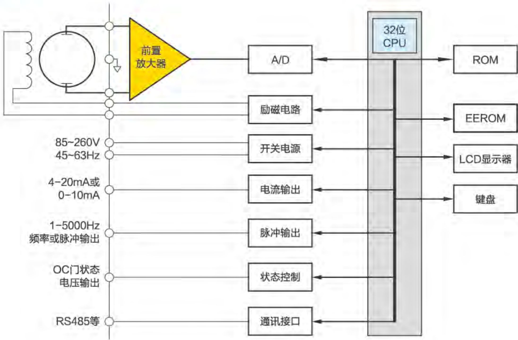
电磁流量计电路结构图
