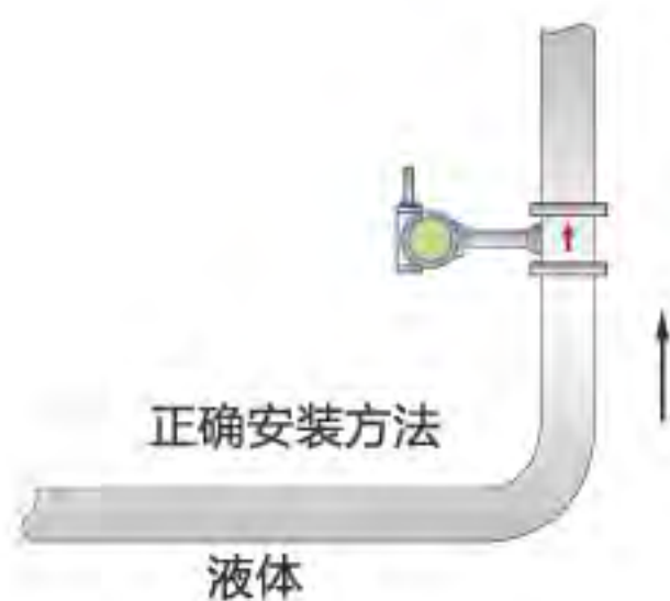
图三 液体管道安装
