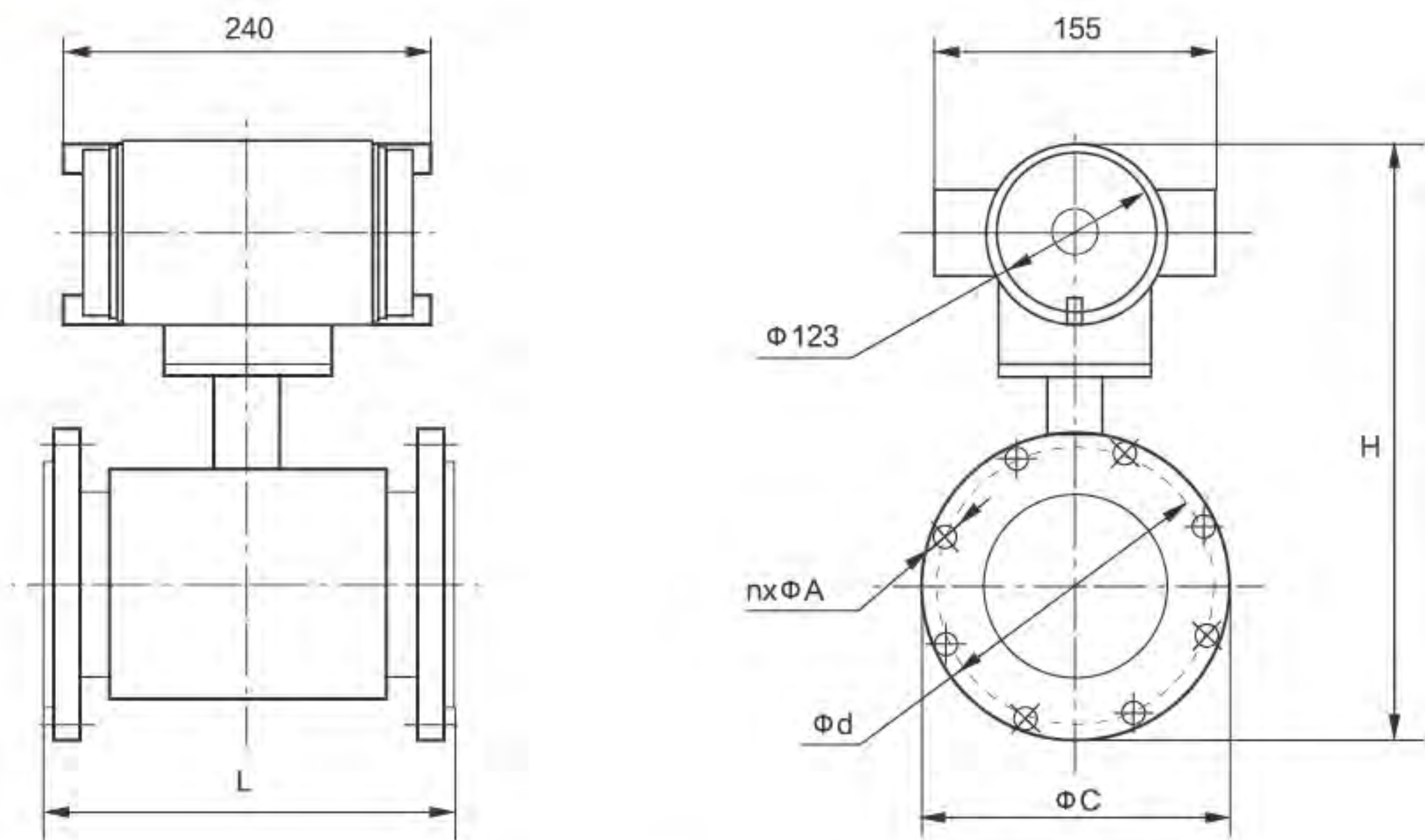
LDQL电磁流量计外形示意图
