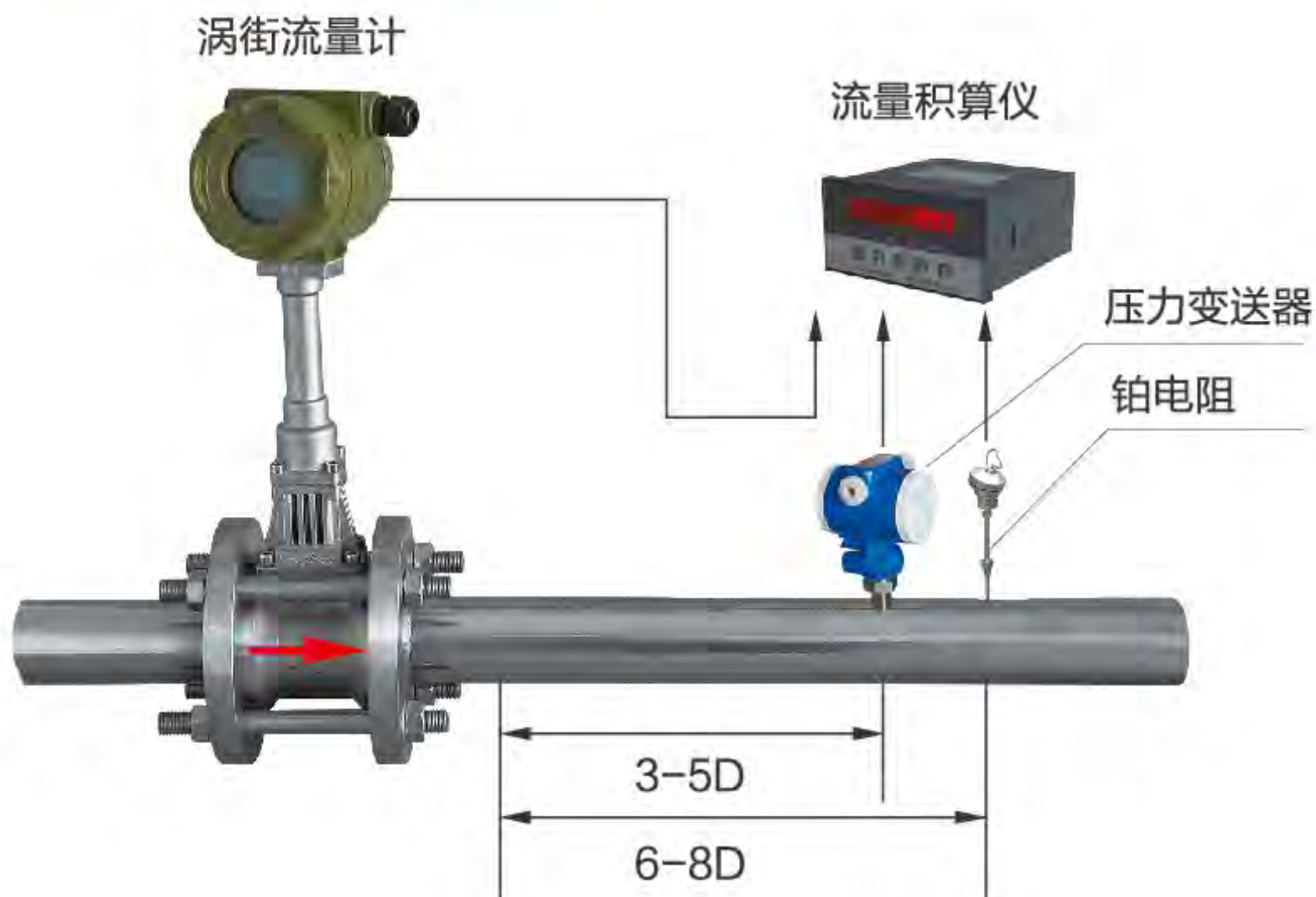
图五 取压点和测温点位置图
