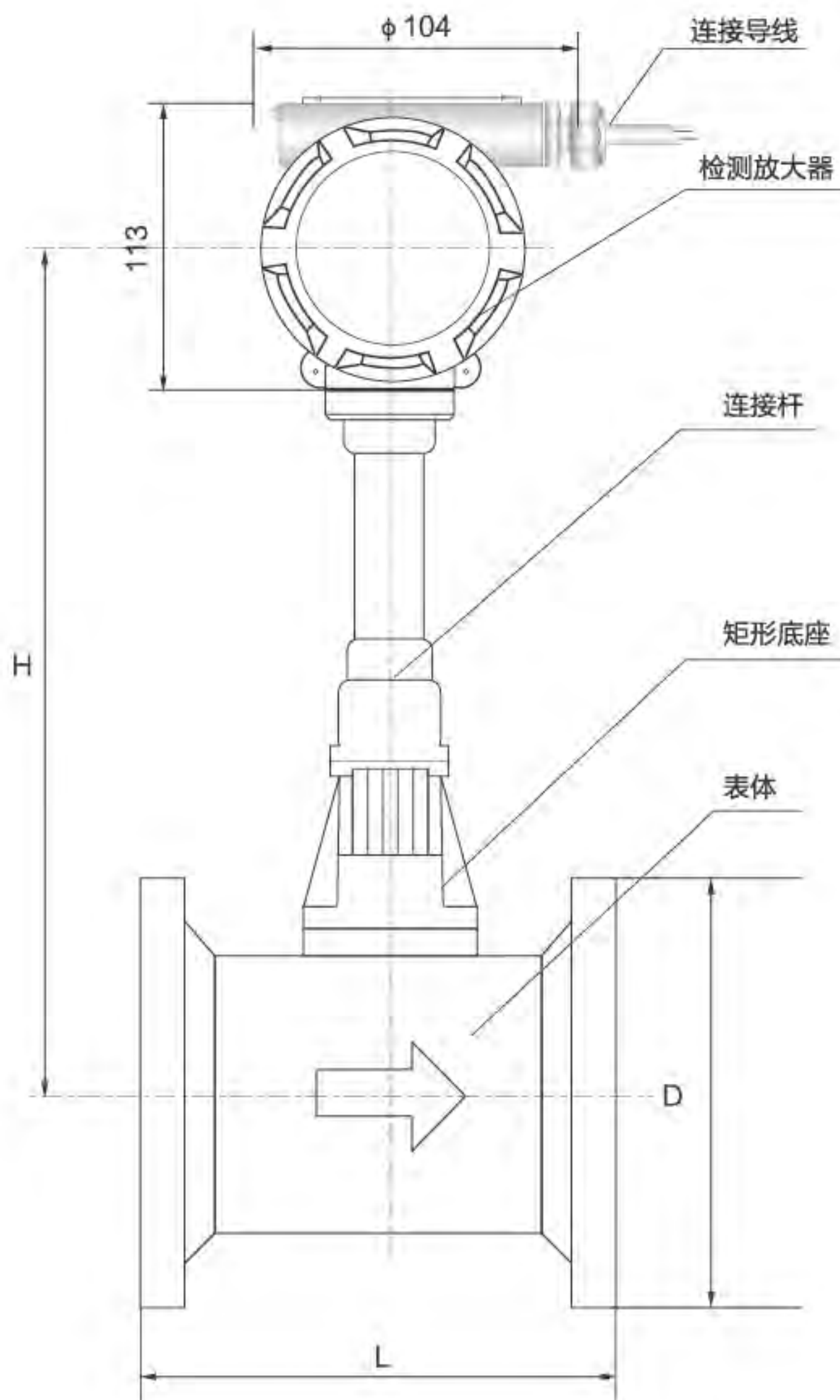
图一 LUGB型涡街流量计外形尺寸
