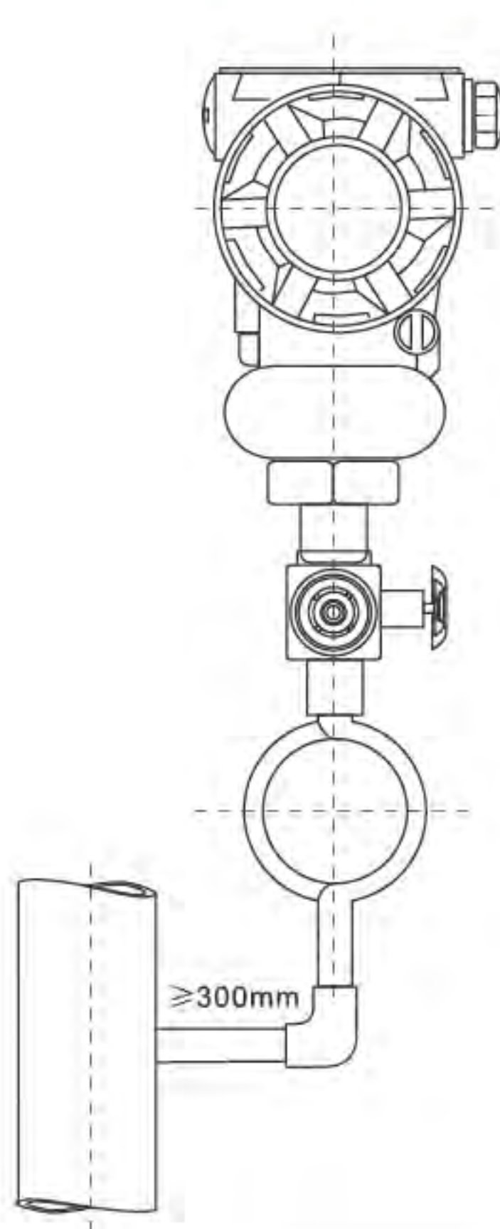
图3 (b) 立式安装方式
