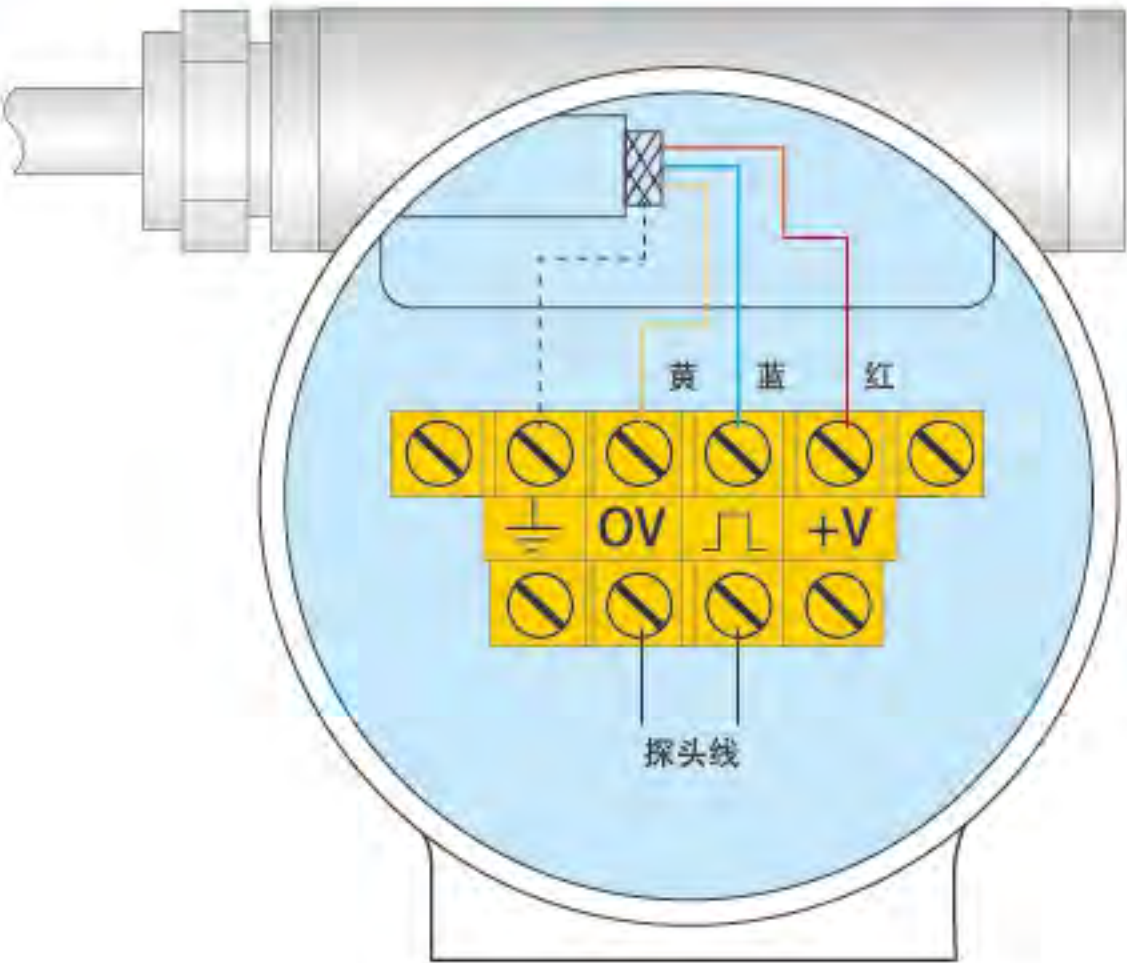
图六 屏蔽电缆接线位置
