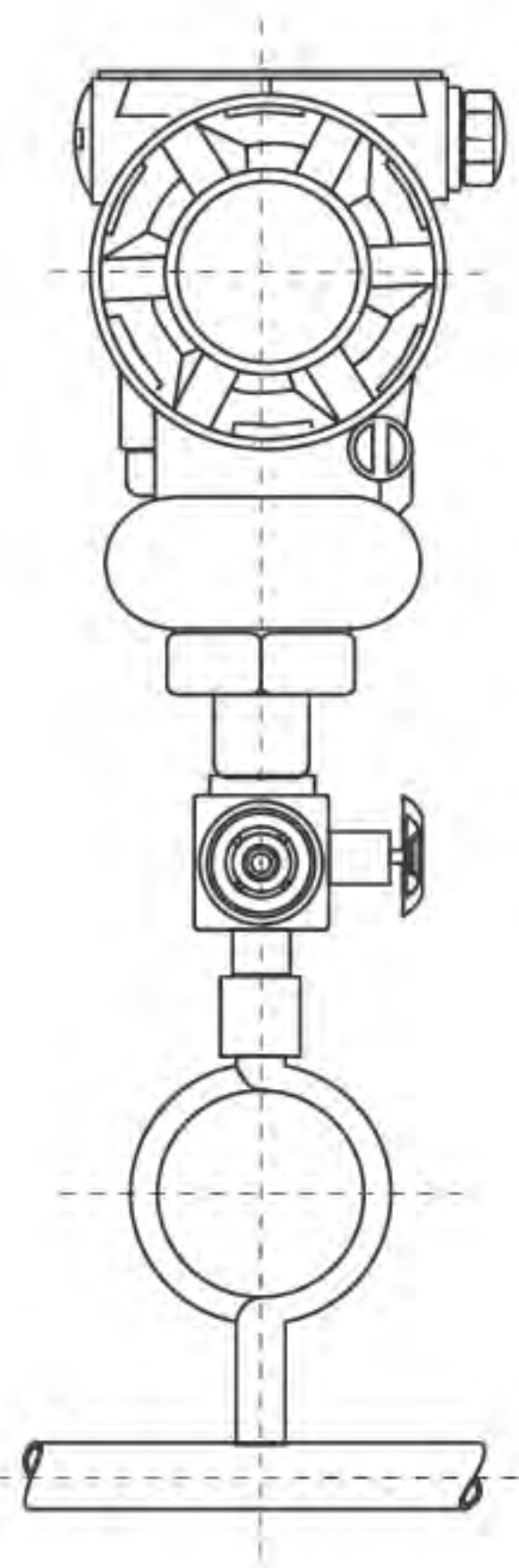
图3 (a) 水平安装方式
