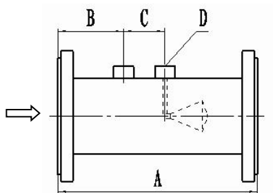
法兰连接式 (LVQLS) 外形尺寸表
