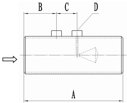
直接焊接式 (LVQLZ) 外形尺寸表
